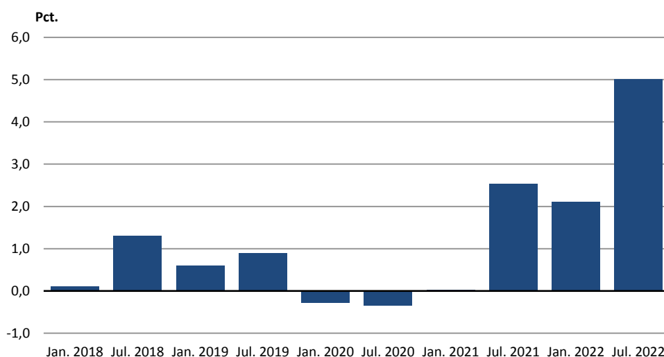
Figur 1. Byggeomkostningsindekset halvårslige ændringer, januar 2018 – juli 2022
